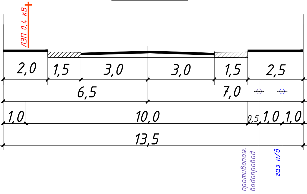
Разрез 1-1
